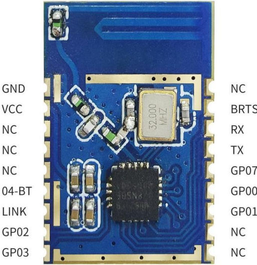
图 1-模块引脚图
