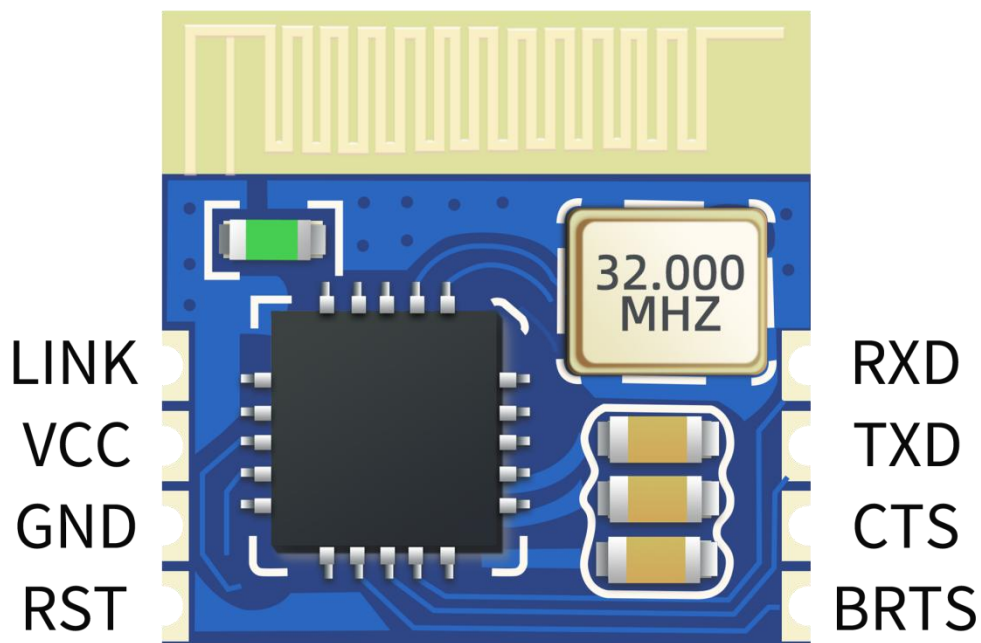
图 1-模块引脚图
